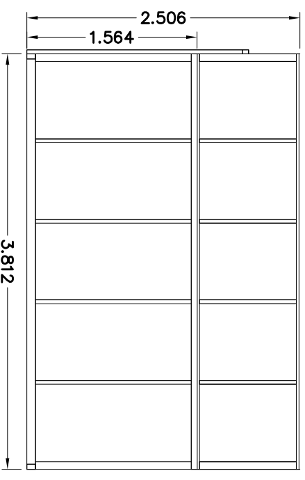
AANZICHT B
