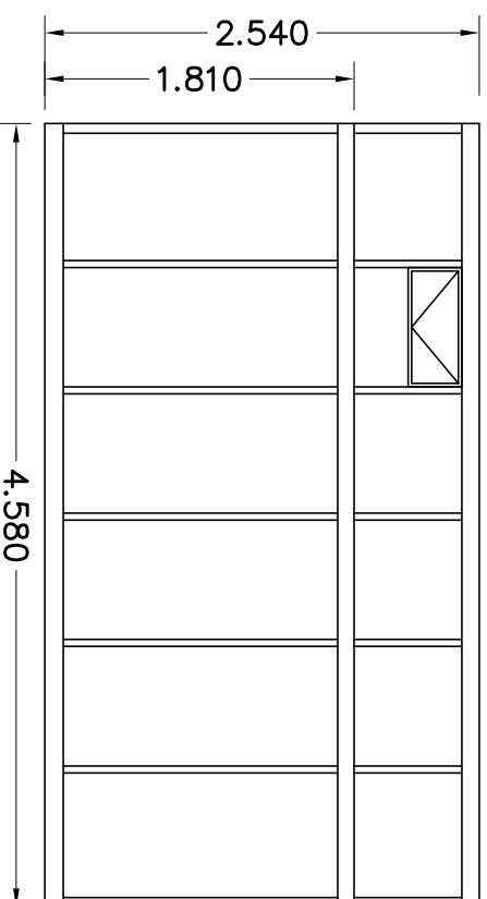
AANZICHT B
