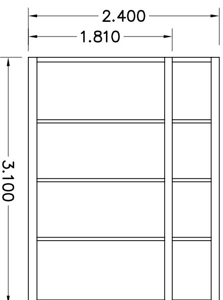
AANZICHT B
