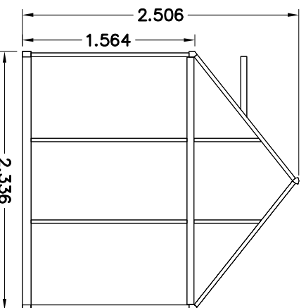
AANZICHT C
