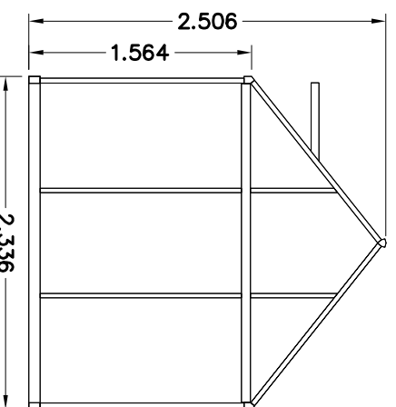
AANZICHT C
