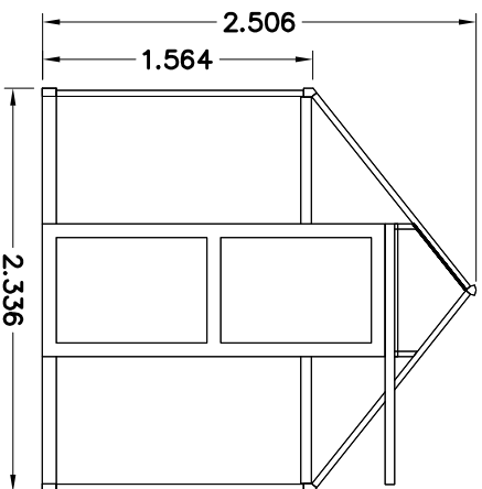
AANZICHT A
