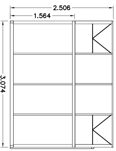
AANZICHT D
