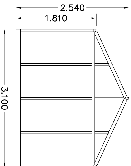
AANZICHT C
